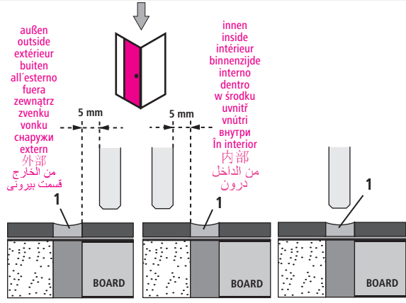
2 Versiegelung / Sealing / Scellement / Siliconen-kitnaad / Sigillatura Sellado / Uszczelnienie zewnętrzne / Utzavirači nátěr / Tesniaca hmota 3 Zementfuge / Cement joint / Joint en ciment / Cementvoeg / Fuga di cemento Junta de cemento / Spoina cementowa / Cementová spára / Cementová medzera Цементный шов / Rosturi ciment / 水泥缝 / المفصل الأسمنتي / درز سیمان
